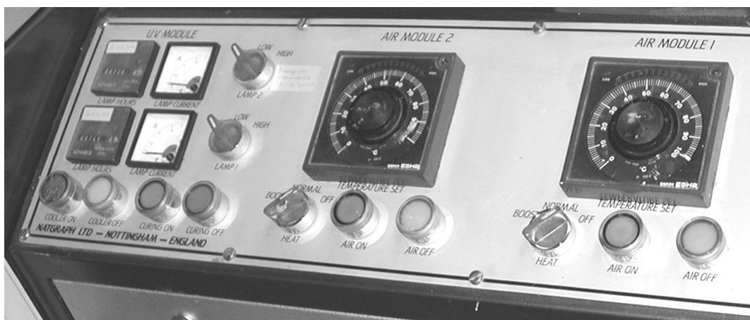
Figuur 2.1: Schakelpaneel van een combi-tunnel, bestaande uit 2 warmelucht-secties en 2 UV-stralers. Het vermogen van de stralers wordt aangegeven op de 2 (witte) Ampèremeters. Rechts daarnaast de instelknoppen voor het lampvermogen, die de standen LOW of HIGH kennen. De grote zwarte temperatuurregelaars behoren bij de twee warmelucht secties.
