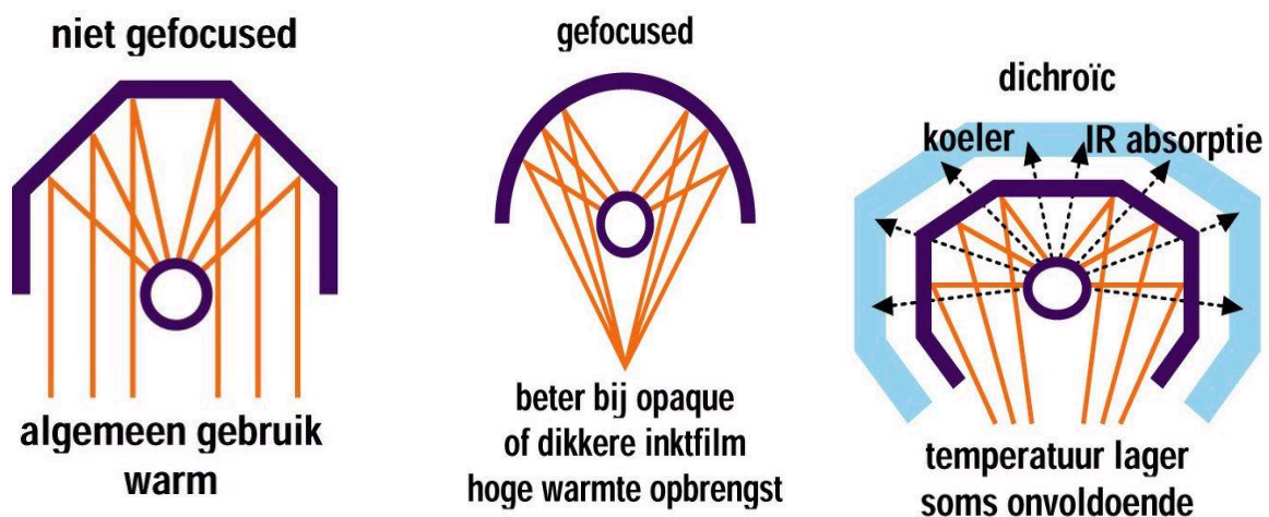
Figuur 3.5: effecten van de reflectorvorm op de droging van UV-inkt
