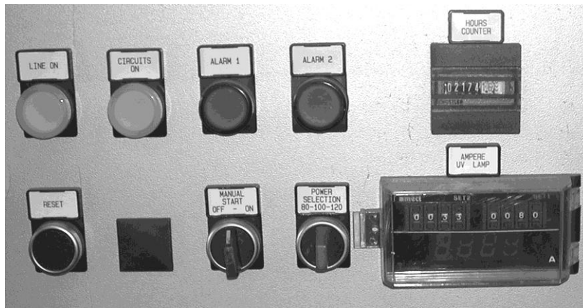
Figuur 3.6: Schakelpaneel van een éénlamp 100% UV-tunnel. De vermogensschakelaar van de UV-lamp (POWER) SELECTION kent de standen 80, 100 en 120 W/cm. Er is voorzien in een Ampèremeter (AMPERE UV-LAMP), hetgeen een indicatie geeft van het lampvermogen. Tevens is een brandurenteller (HOURS COUNTER) ingebouwd.
