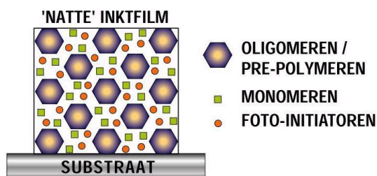
Figuur 3.2: Curing van UV-inkten onder invloed van UV-straling (zie figuren a,b en c)
