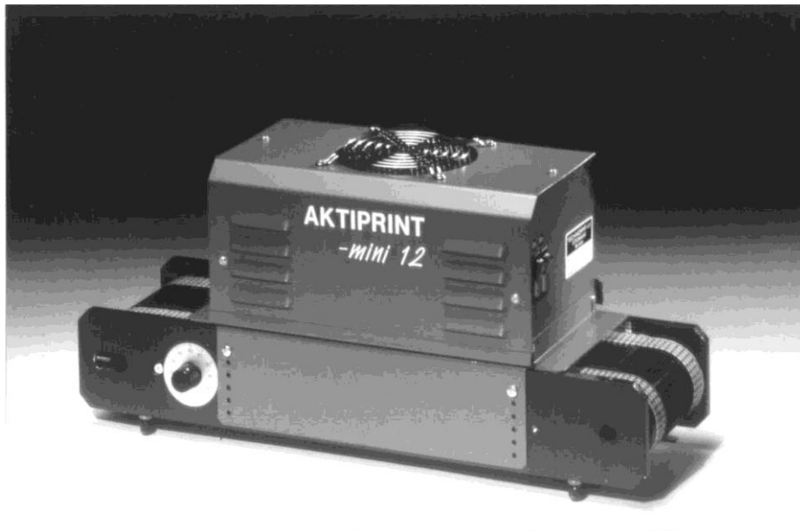
Figuur 4.2: Een laboratorium UV-droger leent zich uitermate goed voor het uitvoeren van testen, ter beoordeling van curing en hechting. Deze UV-droger kan in 12 cm en 18 cm stralerbreedte worden uitgevoerd, zowel in éénlamps als tweelamps uitvoering.
